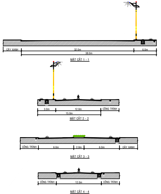
MẶT CẮT NGANG ĐIỂN HÌNH SÀN ĐƯỜNG NỘI BỘ
