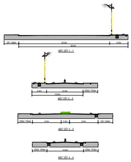
MẶT CẮT NGANG ĐIỂN HÌNH SÂN ĐƯỜNG NỘI BỘ
