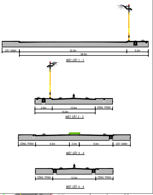
MẶT CẮT NGANG ĐIỂN HÌNH SÂN ĐƯỜNG NỘI BỘ
